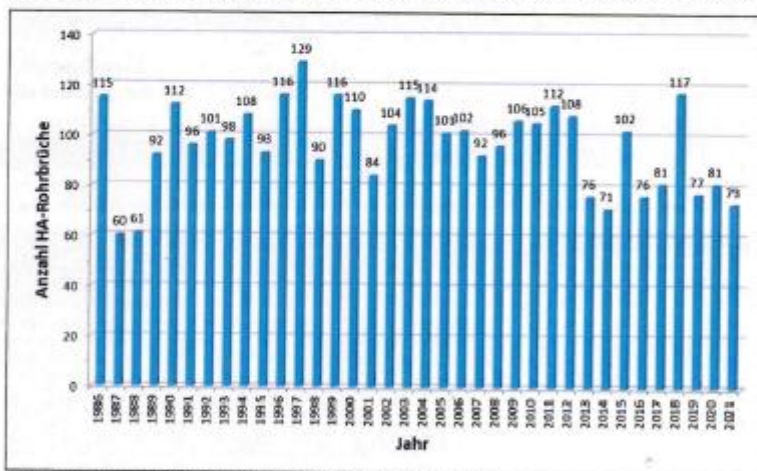
Anzahl der Rohrbrüche pro Jahr im Hausanschlussbereich.
