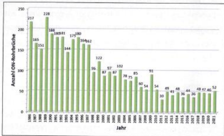
Anzahl der Rohrbrüche pro Jahr im Verteilungsnetz.
